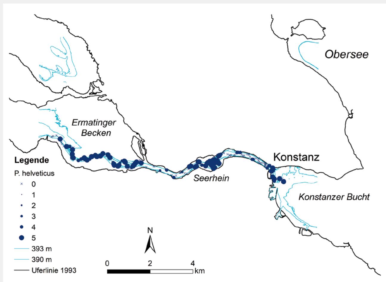
Fig. 3 Ergebnisse der Kartierung der immergrünen Bestände des Schweizer Laichkrauts ( Potamogeton helveticus ) von der Konstanzer Bucht im Obersee über den Seerhein bis ins Ermatinger Becken des Untersees am 15. und 16. März 2017. Die Pflanzenmengenangaben beziehen sich auf die Skala nach [16]: 1 = sehr selten, 2 = selten, 3 = verbreitet, 4 = häufig, 5 = massenhaft.
