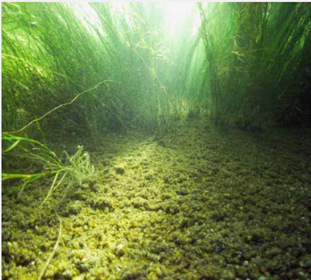
Fig. 4 Sprossdichten des Schweizer Laichkrauts in der Fliessrinne beim Inselhotel in Konstanz.
