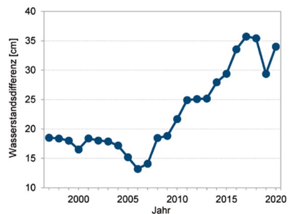
Fig. 1 Verlauf der Wasserstands-differenz zwischen dem Obersee (Pegel Konstanz) und dem Untersee (Pegel Radolfzell) über 24 Jahre. Die verwendeten Bezugsniveaus der Pegel waren: 391.895 m ü. NN für den Pegel Konstanz und 391.894 m ü. NN für den Pegel Radolfzell (Höhensystem DHHN92 [HS 160]). (Datenquelle: LUBW)
