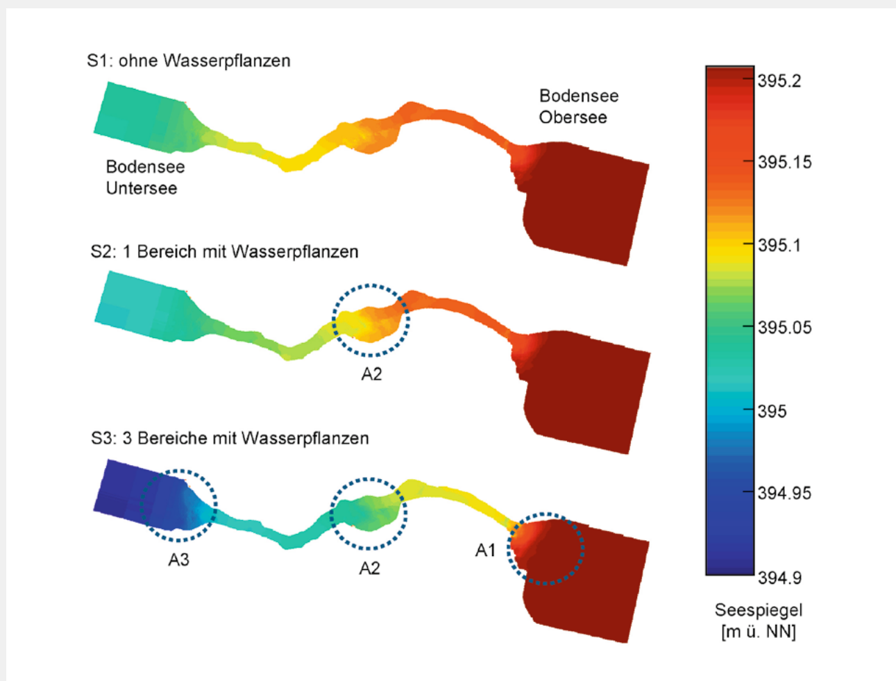
Fig. 5 Darstellung der berechneten Wasserstände zwischen dem Obersee (rechts) und dem Untersee (links) für die drei Modellszenarien S1 bis S3. Die Kreise geben grob die Lage der Wasserpflanzenbereiche A1 bis A3 an.
