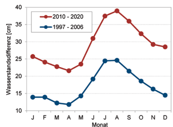
Fig. 2 Höhendifferenz der Wasserstände des Obersees und des Untersees in den einzelnen Monaten über zwei Zeiträume. (Datenquelle: LUBW)
